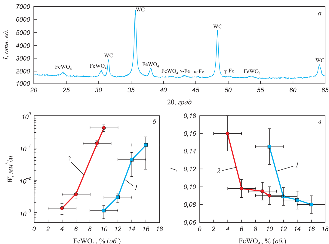
Рис. 2. Рентгенограмма изношенной поверхности WC – 80Г4 после скорости скольжения 37 м/с (а), зависимости интенсивности изнашивания W (б) и коэффициента трения f (в) от содержания \text{FeWO}_4 на изношенной поверхности композитов WC – 80Г4 (1) и WC – 80Г20 (2)
