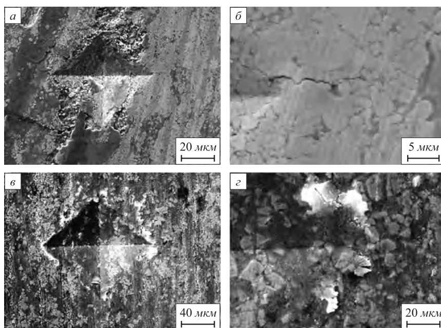
Рис. 3. Изображения РЭМ отпечатков индентора Виккерса на поверхности трения композита WC – 80Г4: после трения при скорости 20 м/с (а, б); после трения при скорости 37 м/с (в, г)
