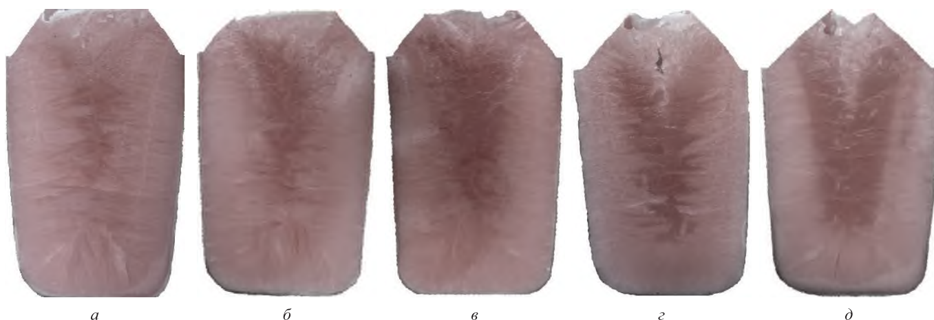
Рис. 4. Макроструктура модельных слитков, отлитых при различных скоростях разливки расплава сверху и сифоном: а – массовая скорость разливки расплава сверху 20 г/с ( D_{ст} = 3 мм); б – массовая скорость разливки расплава сверху 51 г/с ( D_{ст} = 11 мм); в – массовая скорость разливки расплава сверху 72 г/с ( D_{ст} = 18 мм); г – массовая скорость разливки расплава сифоном 5 г/с ( D_{ст} = 3 мм); д – массовая скорость разливки расплава сифоном 7,5 г/с ( D_{ст} = 6 мм)
