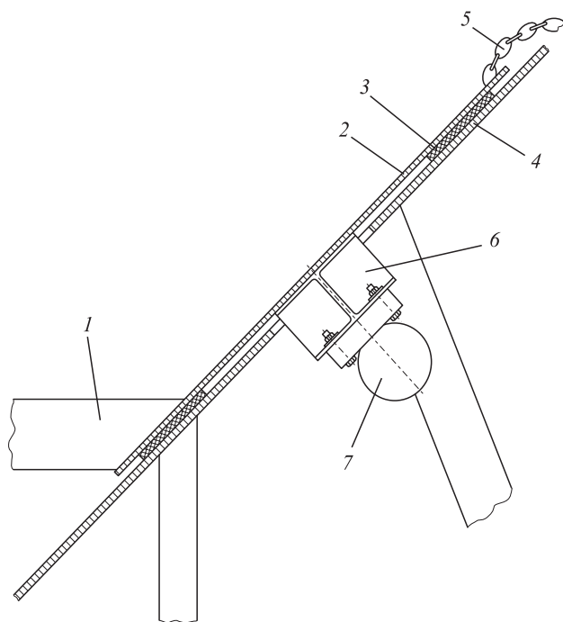
Рис. 2. Вибрационное устройство «ложная стенка»: 1 – вибрирующая балка (виброгорбыль); 2 – плита (ложная стенка); 3 – амортизатор (транспортная лента); 4 – стенка бункера; 5 – цепь; 6 – опора вибратора; 7 – вибратор
