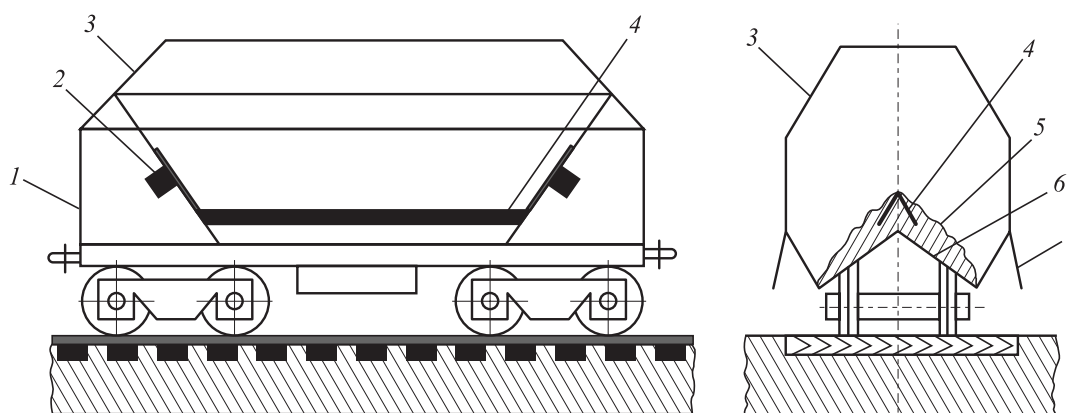
Рис. 1. Схема вагона-хоппера после модернизации: 1 – корпус; 2 – вибратор; 3 – бункер; 4 – вибрирующая балка (виброгорбыль); 5 – сводообразование агломерата; 6 – хребтовая балка; 7 – разгрузочный люк
